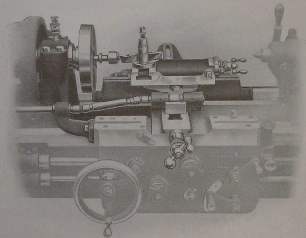
End relief
